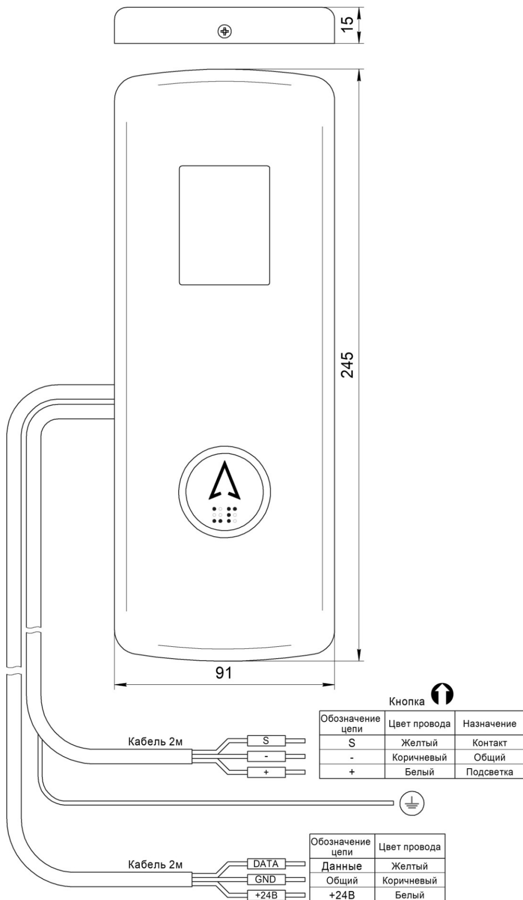
Рис.1 Внешний вид, габаритные и установочные размеры Вызывного поста ЦИРКОН НШЕК.468381.078
